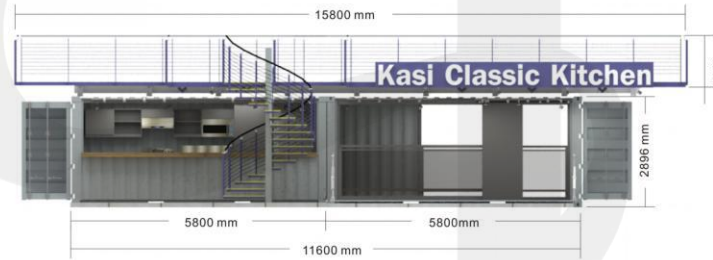
A Elevation
