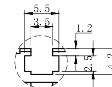
视图C, 比例2:1
