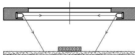
照明示意图
