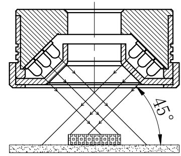
照明示意图
