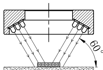
照明示意图
