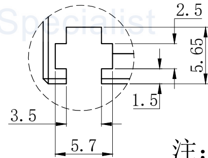
视图A 比例2:1
