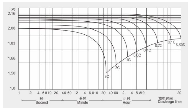
图-4 自放电特性及补充充电方法
